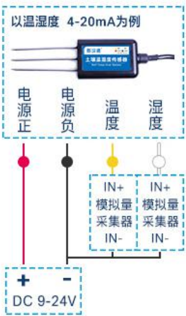
■ 两参数模拟量接线说明
