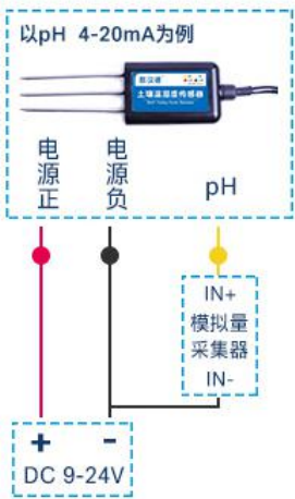
■ 单参数模拟量接线说明
